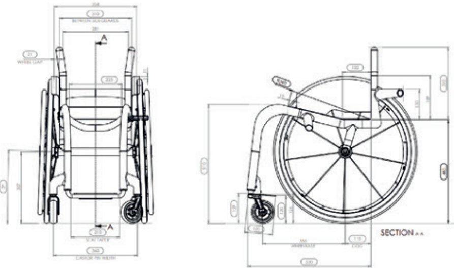
DIBUJO CAD DE LA SILLA VEYPR SUB4 DE DAVID
