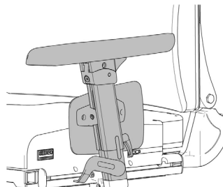
Reposabrazos desmontables // QOP040021
