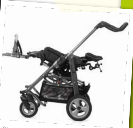
Sistema BSS que mantiene el centro de gravedad durante la basculación
