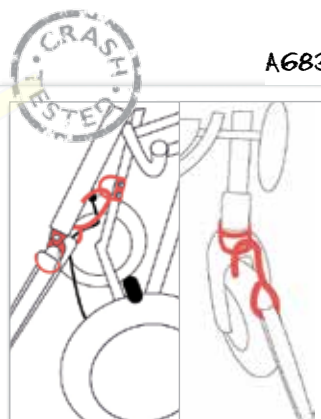
Anclaje para el transporte en vehículos
